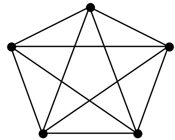
K_5
