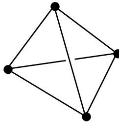
K_4
