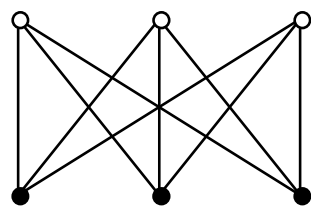
K_{3,3}
