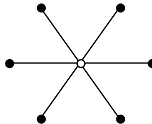
K_{1,6}
